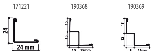
L-randafwerkingsprofiel 24x24 mm
